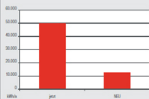
Energieverbrauch für Heizung: Standort Kläranlage Stegaurach
